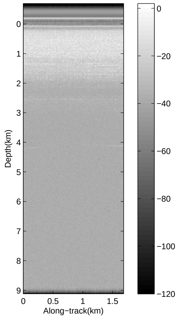
Radar Echogram: Dec08_145-145HG
